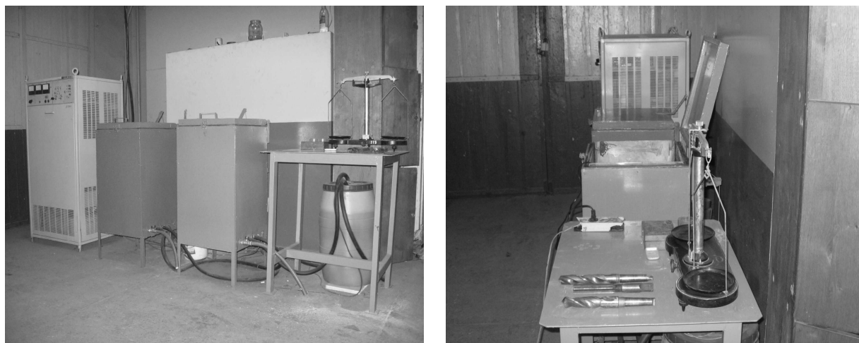
Рис. 9. Установка для комплексной ультразвуковой обработки осевых лезвийных инструментов
