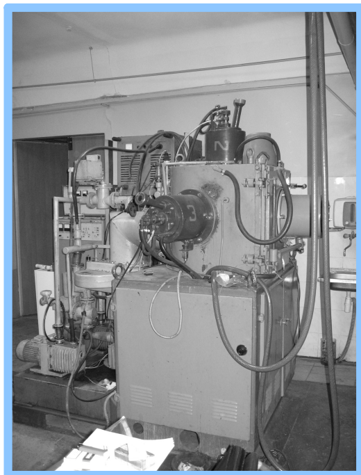
Рис. 10. Общий вид установки ННВ 6.6-II1 для вакуумного ионно-плазменного напыления покрытий на лезвийный инструмент
