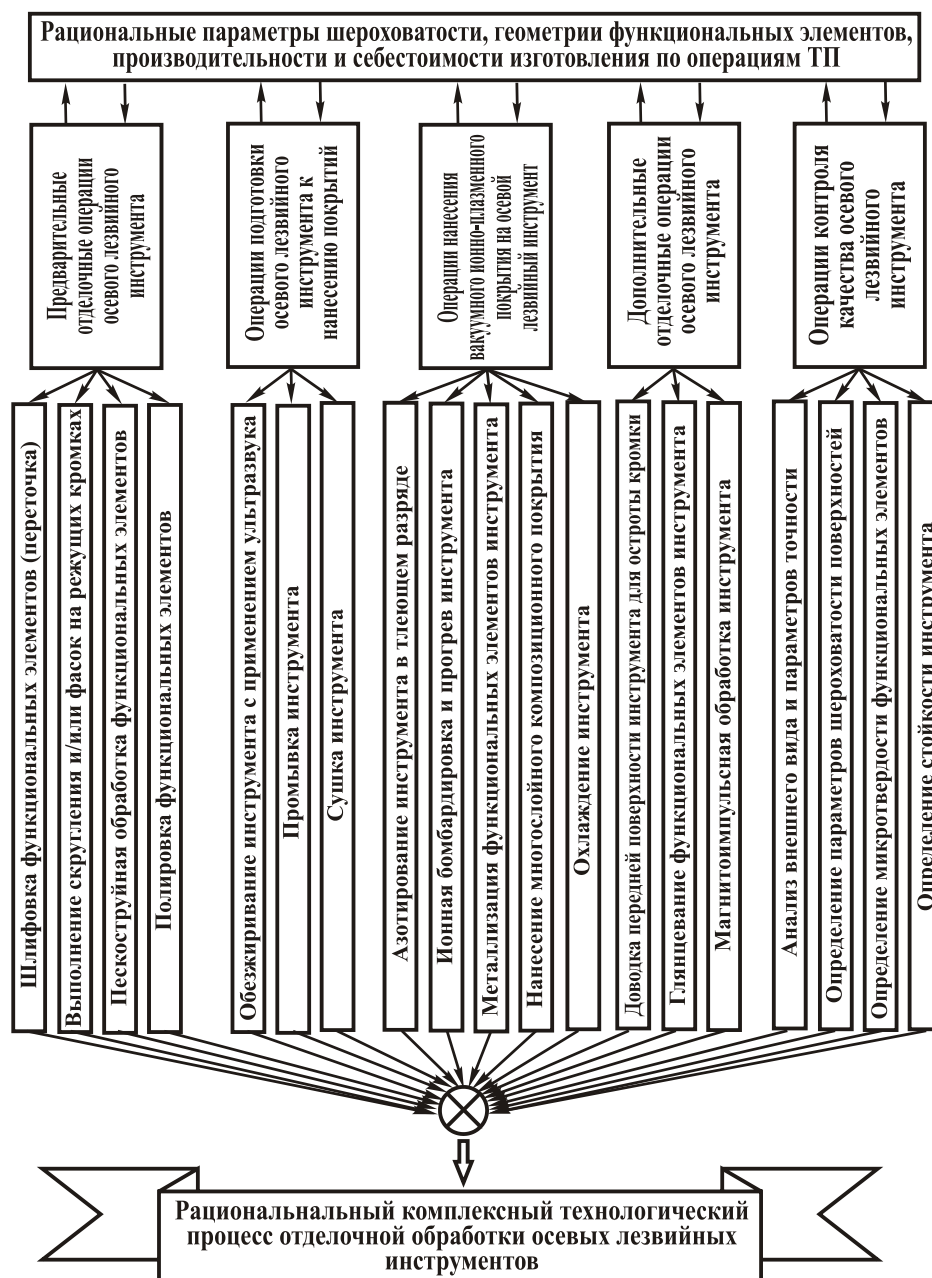
Рис. 4. Иерархическая схема структуры рационального технологического процесса дополнительной отделочной обработки осевых лезвийных инструментов
