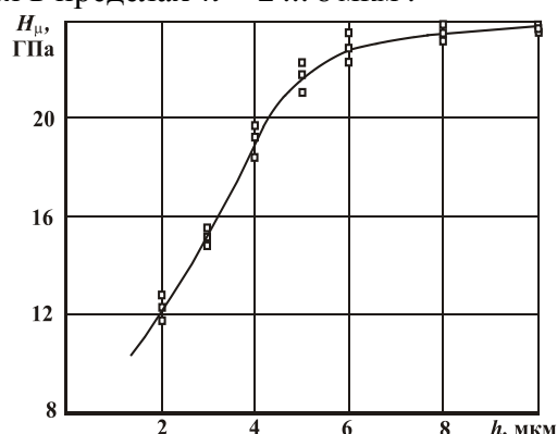
Рис. 13. Зависимость микротвердости нитрид титанового TiN покрытия от его толщины (материал подложки - сталь инструментальная легированная ХВ4Ф, исходная микротвердость -(0,3 - 0,4) \cdot 10^3 МПа, исходная шероховатость - R_{a1} = 0,080 мкм)
