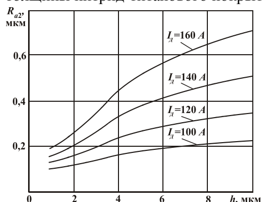
Рис. 12. Зависимость шероховатости поверхности R_{a2} инструмента с нитрид титановым покрытием TiN от его толщины h для различных параметров тока дуги I_d (материал подложки - сталь инструментальная легированная ХВ4Ф, исходная микротвердость -(0,3 - 0,4) \cdot 10^3 МПа, толщина покрытия h = 6 мкм, исходная шероховатость - R_{a1} = 0,080 мкм)
