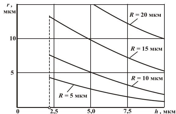
Рис. 15. Зависимость радиуса R закругления режущего клина инструмента (образцов-свидетелей при \beta = 60^\circ ) с нитрид-титановым покрытием от толщины h покрытия и начального радиуса r режущего клина
