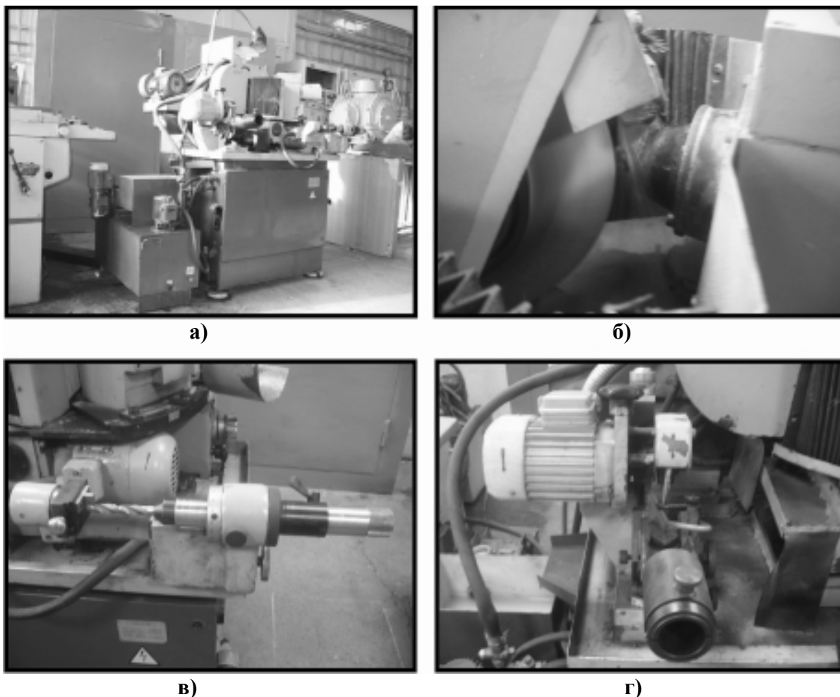
Рис. 5. Общий вид полуавтомата заточного для сверл, зенкеров и метчиков модели 3Е653: а – общий вид полуавтомата с приспособлениями; б – зона затыловки задней поверхности инструмента; в – приспособление для базирования инструмента в патроне; г – механизм подточки поперечной кромки
