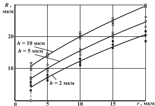
Рис. 14. Зависимость радиуса R закругления режущего клина инструмента (образцов-свидетелей при \beta = 60^\circ ) с нитрид-титановым покрытием толщиной h от начального его радиуса r
