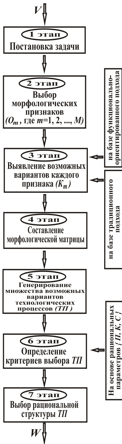
Рис. 3. Основные этапы методики синтеза структуры рационального технологического процесса отделочной обработки осевых лезвийных инструментов
